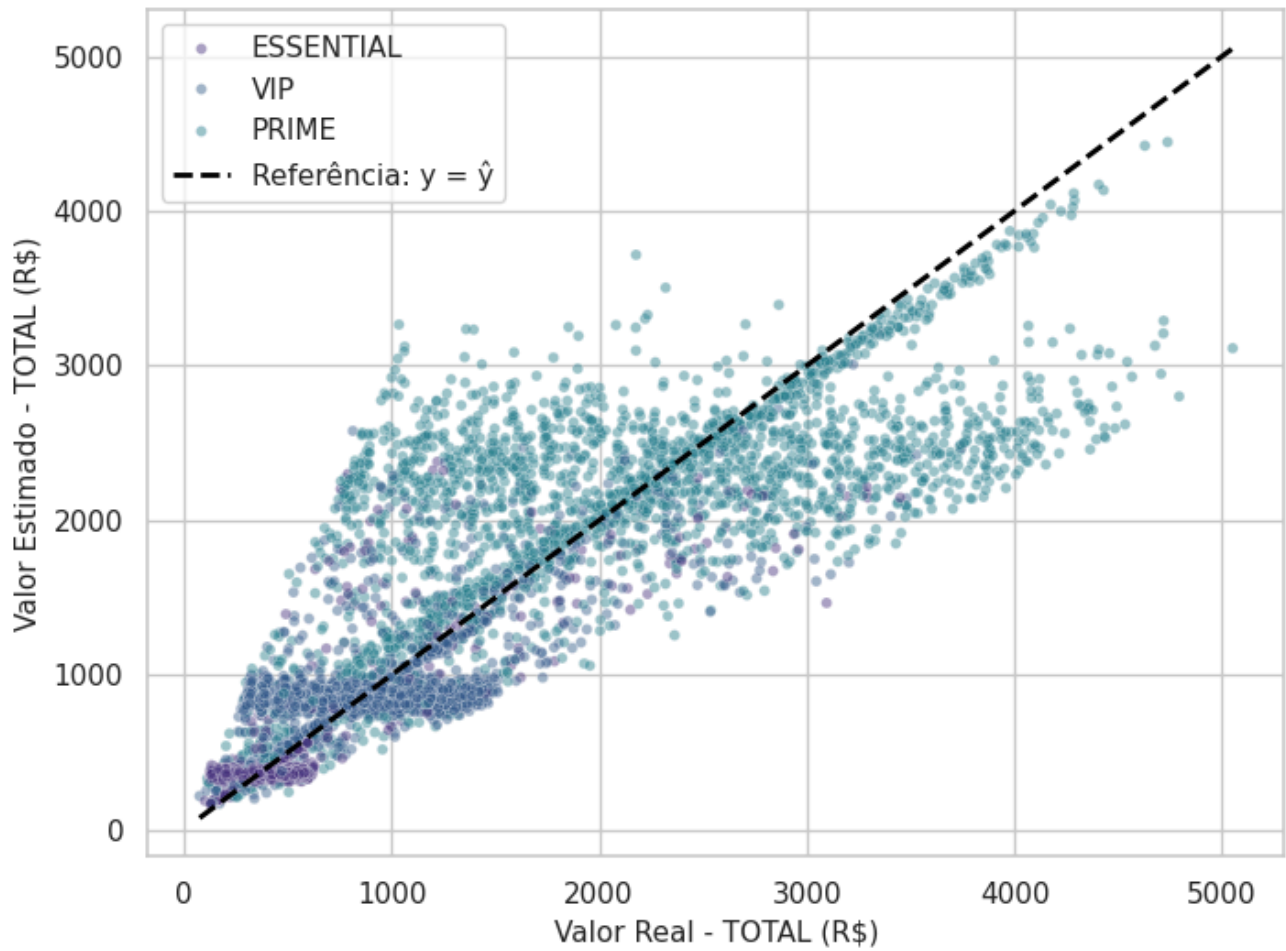
Valores Reais vs Estimados - TEST
