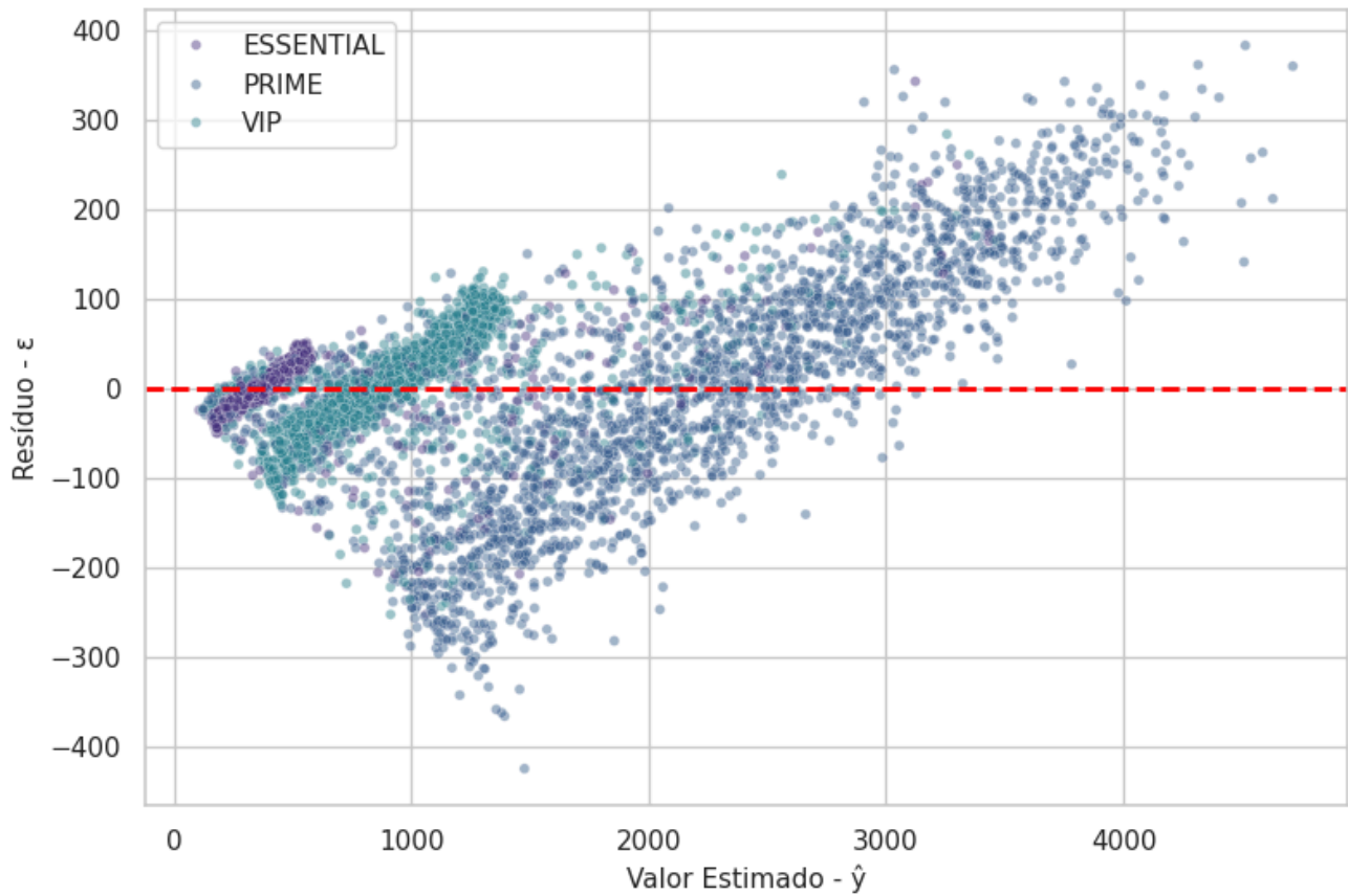
Resíduos vs Valores Estimados - VALIDATION
